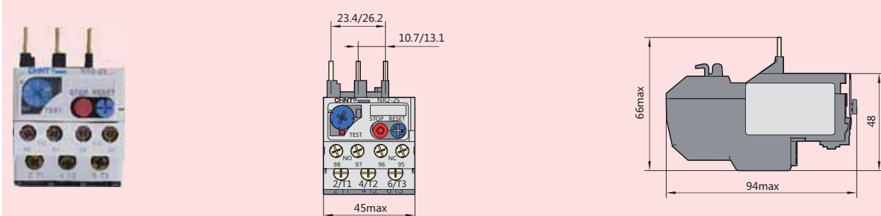
NR2-25外型及安装尺寸
