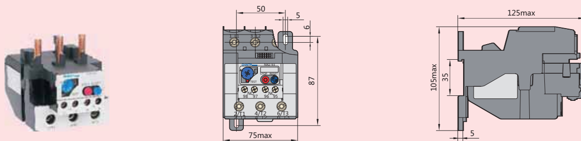
NR2-93带安装座的外型及安装尺寸
