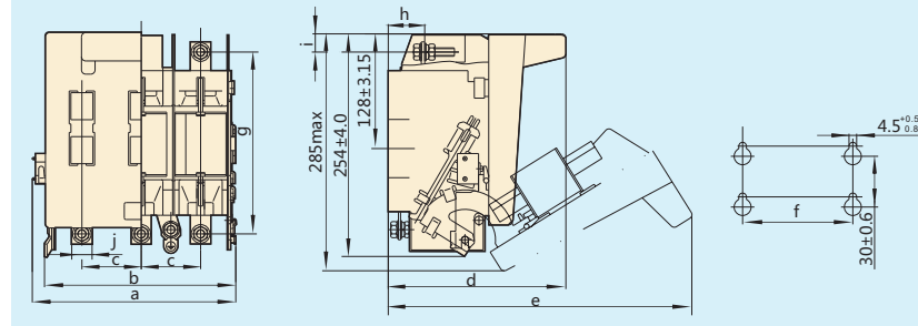
图2 HR5-200-400-630/20、30、31
